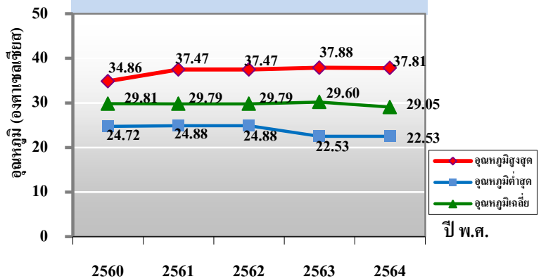
แผนภูมิแสดงอุณหภูมิสูงสุด ต่ำสุด และเฉลี่ยของจังหวัดปทุมธานี ปี 2560-2564
