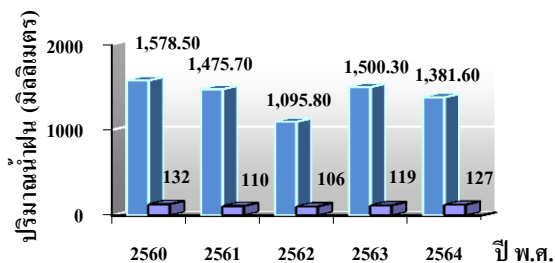
แผนภูมิแสดงปริมาณน้ำฝนและจำนวนวันที่ฝนตกในพื้นที่จังหวัดปทุมธานี ปี 2560-2564
