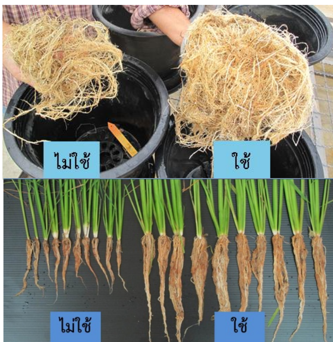
ภาพที่ 7 ผลการใช้ปุ๋ยชีวภาพฟิซีฟิอาร์ต่อการเพิ่มปริมาณรากของข้าวโพด (บน) และข้าว (ล่าง)
