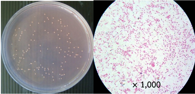
ภาพที่ 3 ลักษณะโคโลนีของแบรคดีไรโซเบียม ( Bradyrhizobium sp.) ที่เจริญบนอาหารเลี้ยงเชื้อ (ซำย) และลักษณะของเซลล์ภายใต้กล้องจุลทรรศน์ (ขวา)
